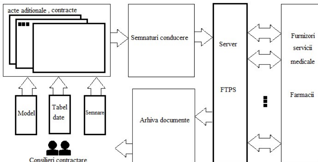
Fig. V. 1 Circuitul documentelor electronice în CAS Iași.
